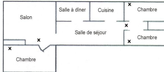
FIGURE 3 : Exemple de localisation des avertisseurs de fumée entre chaque aire où l'on dort et le reste du logement ainsi que dans chaque chambre à coucher
